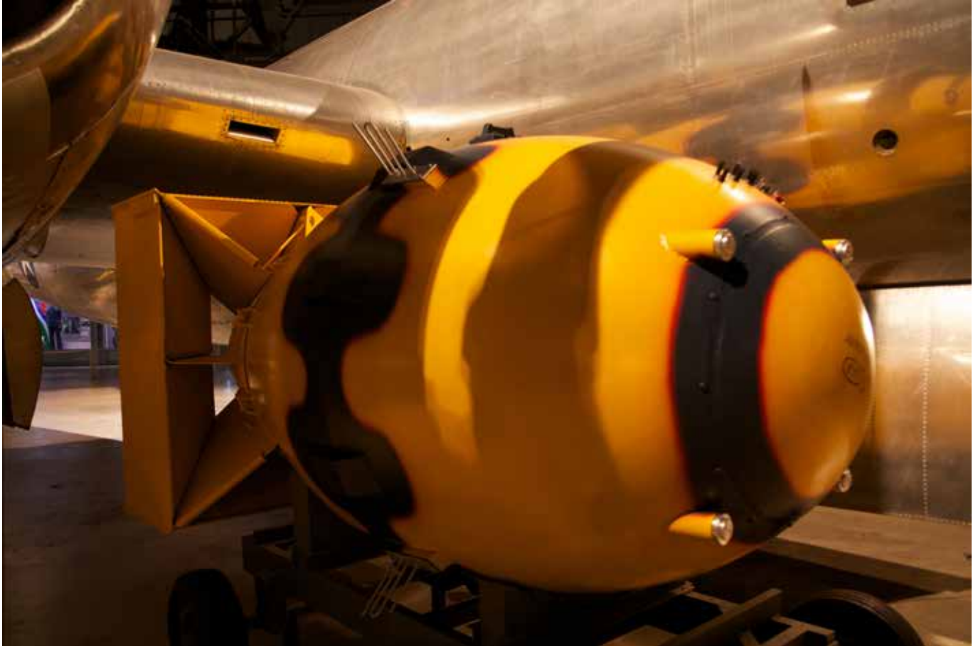
Fat Man på National Museum of the USAF i Dayton, USA. Fat Man var namnet på den typ av atombomb som USA släppte över Nagasaki den 9 augusti 1945. Plutoniumet är omslutet av en sprängladung.
